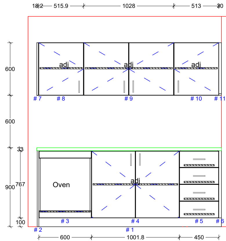
Elevation 1
